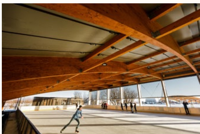
Atklātās publiskās slidotavas segtā jumta izbūve Pasta salā Jelgavā
